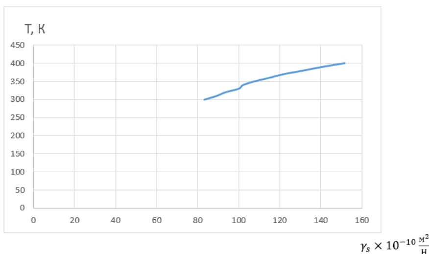
Сызба 1. Авиациялық бензиннің адиабаталық сығылғыштық коэффициентінің температураға тәуелділігі.
