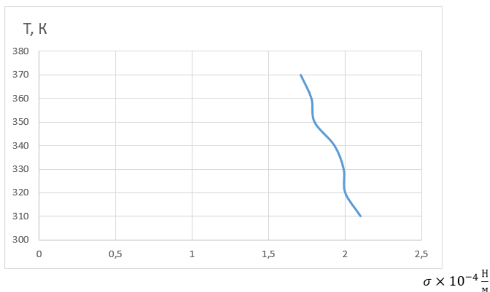
Сызба 2. Этил спиртінің беттік керілу коэффициентінің температураға тәуелділігі.
