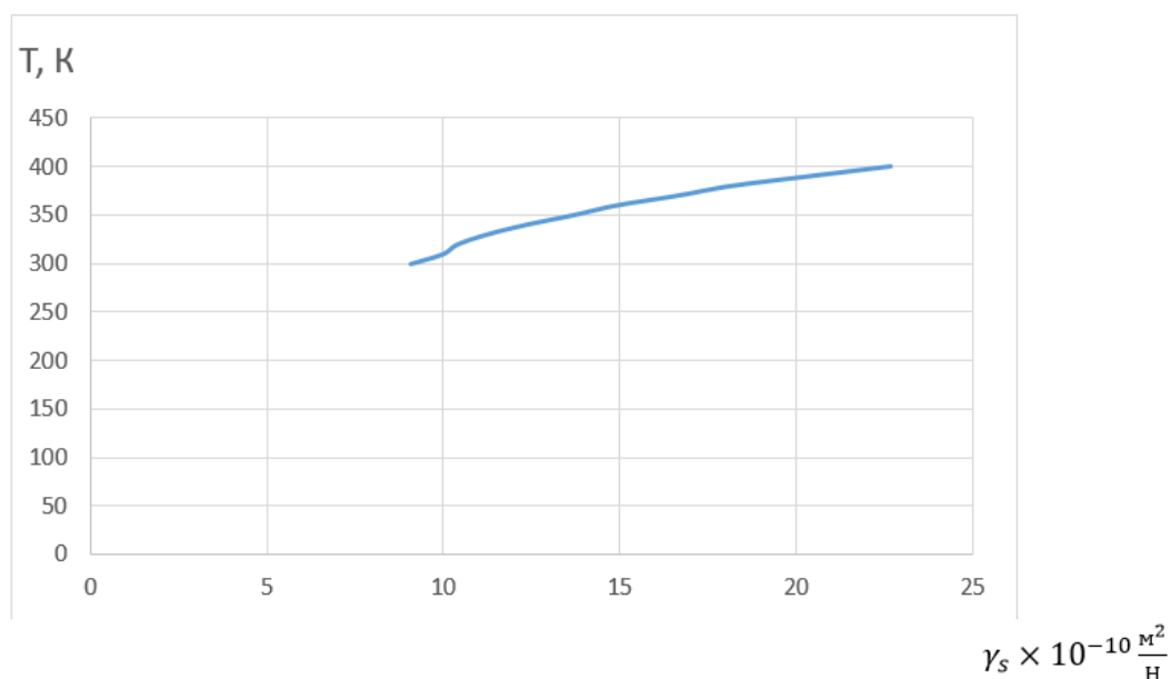
Сызба 1. Мазуттың сығылғыштық коэффициентінің температураға тәуелділігі.
