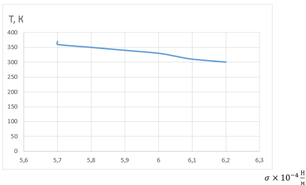
Сызба 1. Глицериннің беттік керілу коэффициентінің температураға тәуелділігі.
